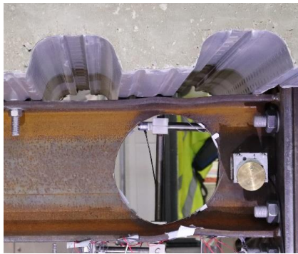
Vierendeel Mechanism.
